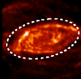
NGC 5055
