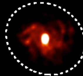
NGC 6946
